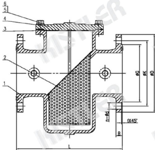
Fig. BS-102 (JIS10K)
